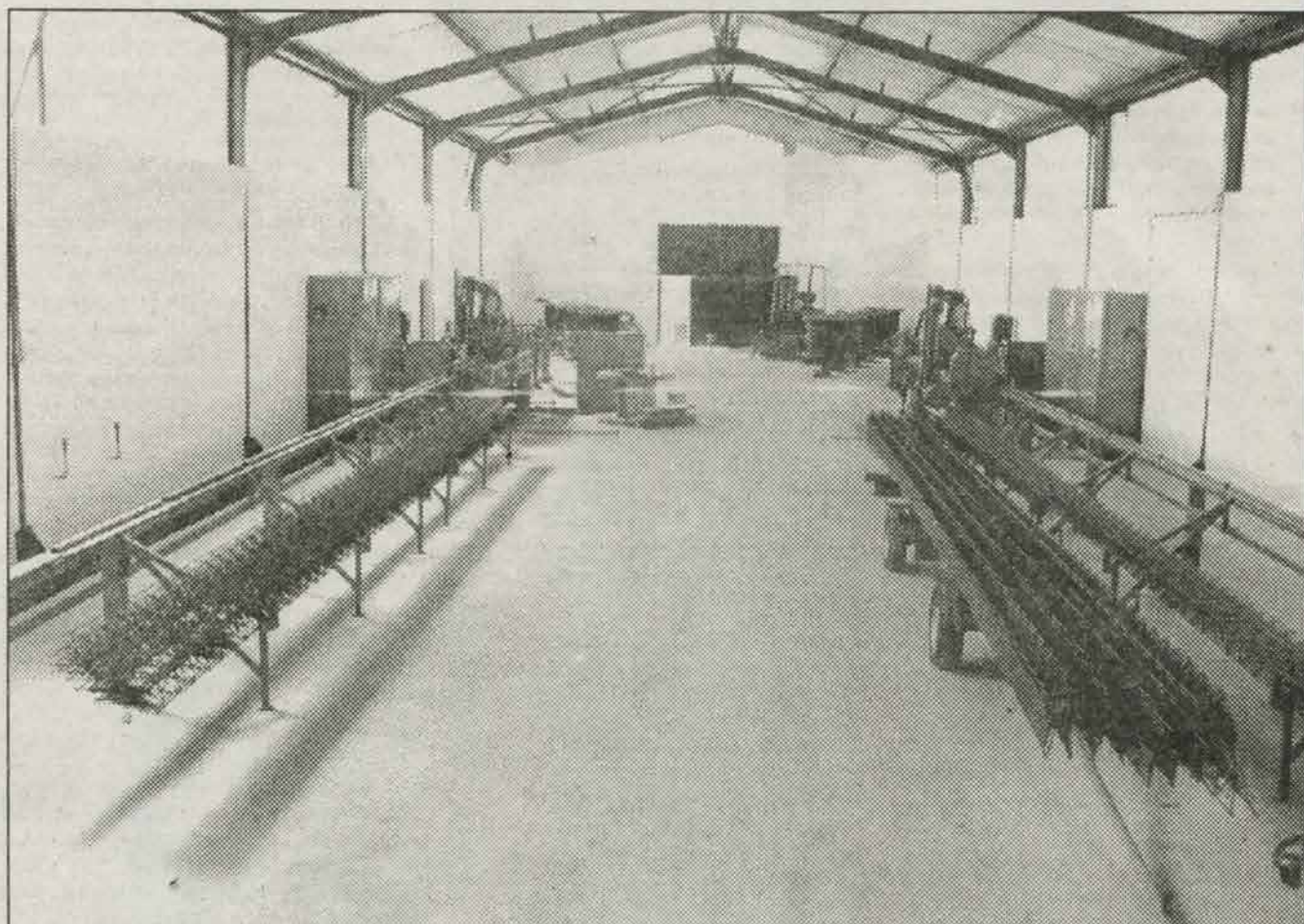
Машине за производњу решеткастих носача увезене из Немачке у периоду санкција
